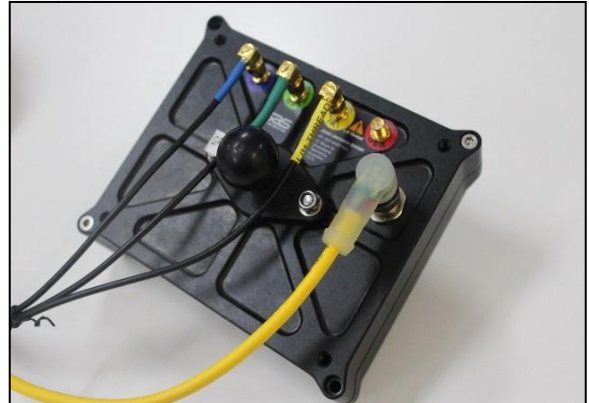
Bild 4: Geräte-Rückseite mit allen Antennen & Stromkabeln verbunden
