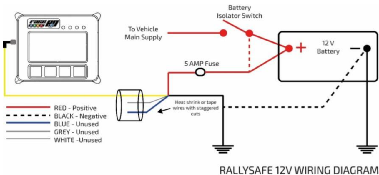
Bild 2: ANSCHLUSS-DIAGRAMM
